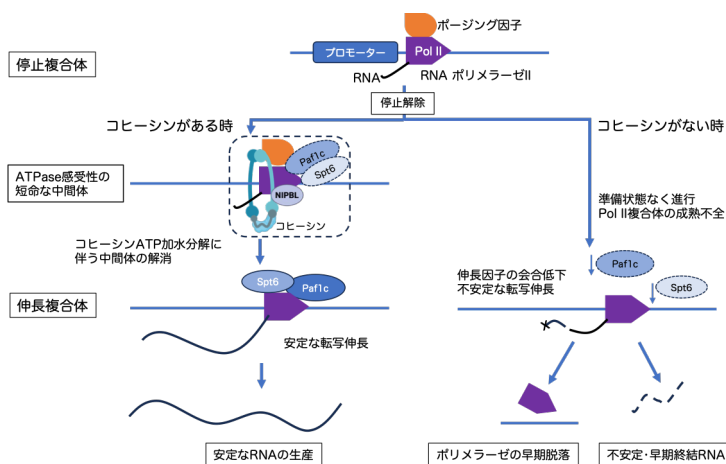
図2：コヒーシンのATPアーゼと同定に成功した短命な転写中間体（点線で囲まれた部分）。CDK9による出発信号の発出直後に、コヒーシンとNIPBLが短時間だけ転写装置へ結合し、PAF1CやSPT6などの補助因子が組み上がる時間を稼ぐという作業モデル。因子同士の直接的な分子接続の解明は、今後の課題となります。
