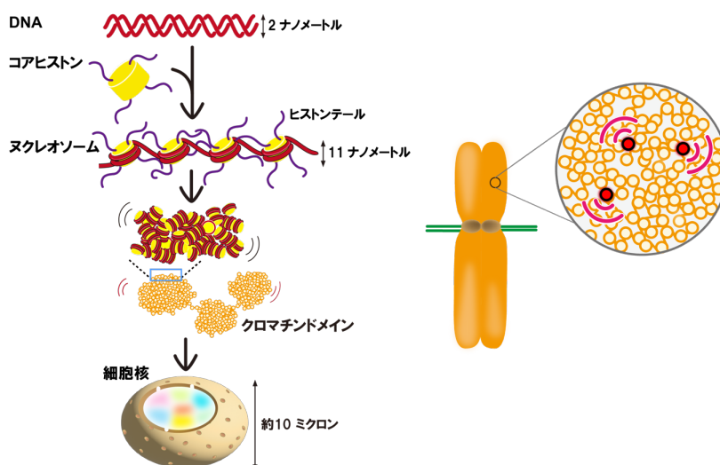
図 1: (左) DNA はヒストンに巻かれてヌクレオソームを形成する。ここでは 4 個のヌクレオソームが描かれているが、1 つの細胞あたり 3000 万個ものヌクレオソームが存在する。ヌクレオソームは不規則に折り畳まれて塊(クロマチドメイン)を形成し、細胞の核のなかに収められている。(右)本研究によって、分裂細胞の染色体のなかの単一のヌクレオソーム(赤)を標識する技術が開発され、その振る舞いが明らかになった。
