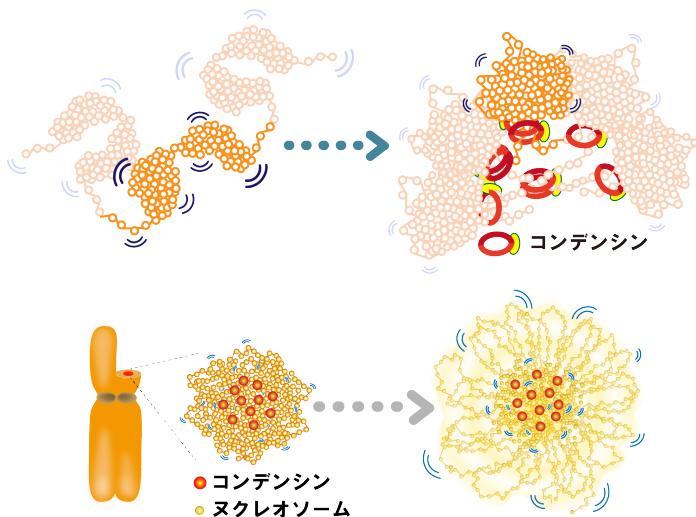
図2: (上段)コンデンシンは、染色体の中心付近でクロマチンドメイン同士を「クリップ」のように結びつけ、ヌクレオソームの揺らぎを抑えている。(下段)ヒストンのテール(尾部)を介したヌクレオソーム間の相互作用を阻害すると染色体が脱凝縮する。ヌクレオソーム間の相互作用も重要な役割を果たしている。
