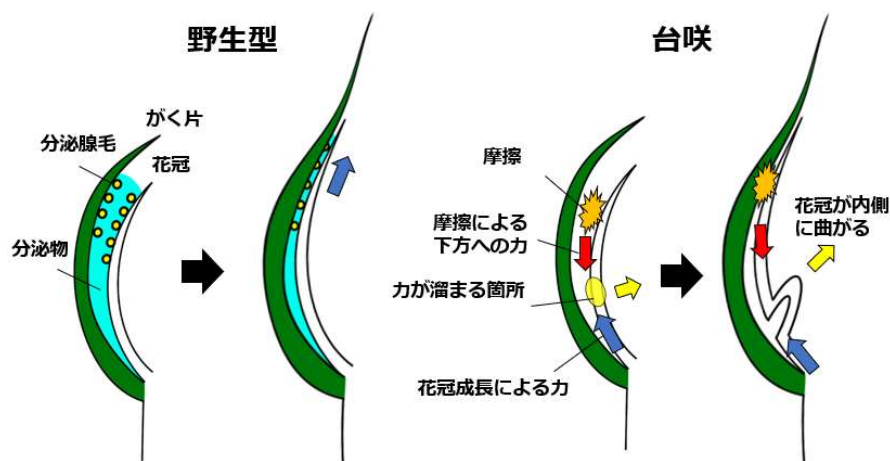
図5 花びら伸長のメカニズム。野生型（左）では分泌腺毛とそこからの分泌物によってまっすぐ伸びる。台咲（右）では分泌腺毛がなく、花びらに摩擦が生じ、曲がってしまう。
