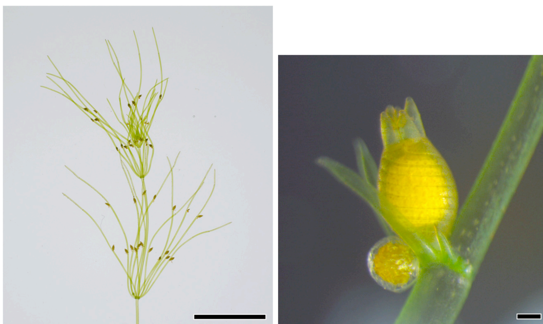
図 1. ゲノム解析に用いたシャジクモ S276 株。(左) 主軸に枝が放射状に輪生し、「車軸」のように見える葉状体。スケールバーは 1 cm。(右) 輪生枝の途中に形成される生殖器官。上が生卵器、下が造精器。スケールバーは 100 \mu m。(神戸大学 坂山英俊 提供)
