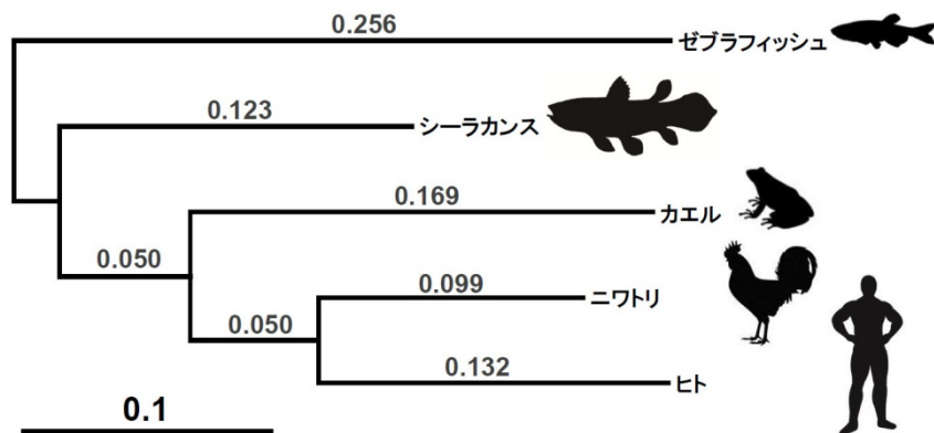
参考図 2: シーラカンスを含めた脊椎動物の系統樹と遺伝子の進化速度。シーラカンスの枝が他生物と比較して顕著に短く、進化速度が遅いことを示している。
