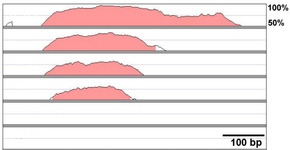
参考図 3: 四肢形成に関わる遺伝子でシーラカンスと四足動物の間で保存された領域。この図では特に bmp7 遺伝子のイントロンに着目。ピンク色に塗りつぶされた領域は種間で保存度が高いことを表す。
