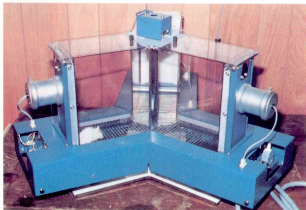
▲ マウスの行動能力を測定するY型迷路自動測定装置
